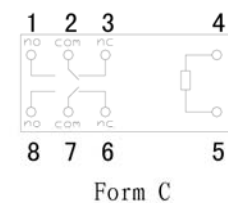
接线图
