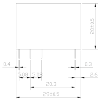
安装图
