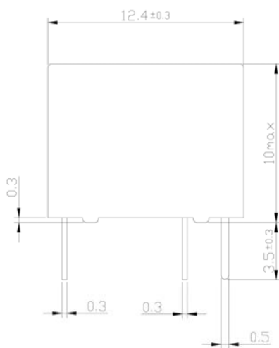
安装图
