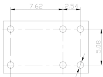
安装图
